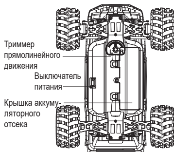
Радиоуправляемый внедорожник
